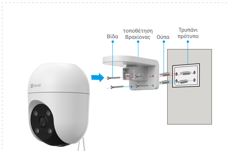
Εικ. 2 Τοποθέτηση στον τοίχο
