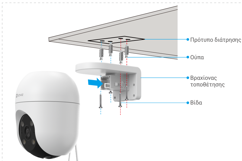
Εικ. 1 Τοποθέτηση στην οροφή
